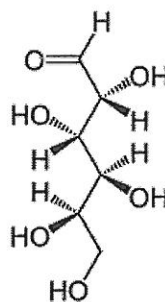
D-galactose
