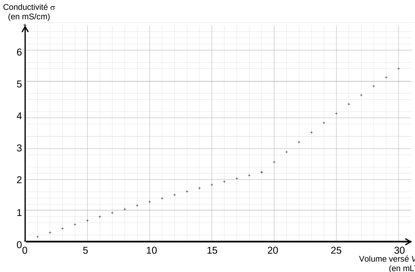
Figure 2 : Évolution de la conductivité \sigma en fonction du volume V de la solution titrante versée
