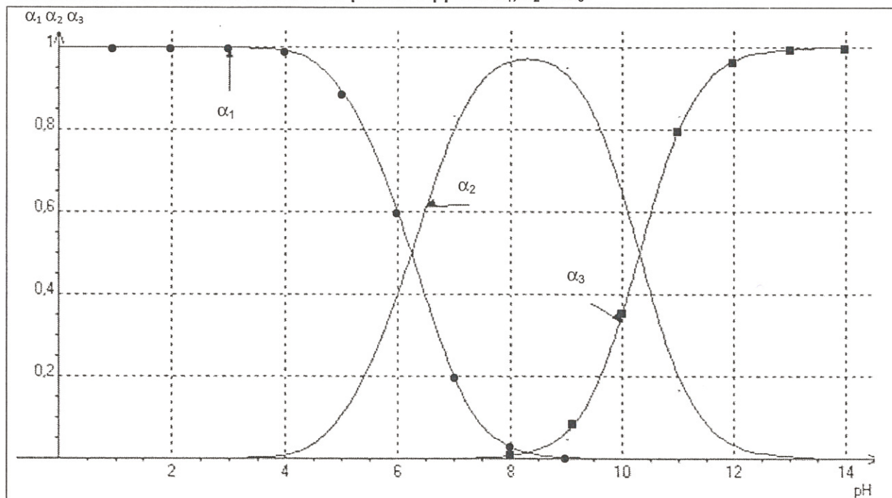
Document 4 - Variation en fonction du pH des rapports \alpha_1 , \alpha_2 et \alpha_3 .
