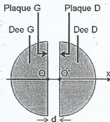
Figure 1. Schéma du cyclotron vu de dessus.
