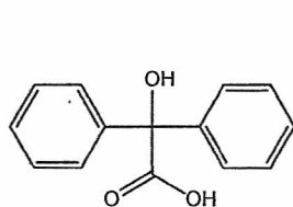
Acide benzylique
