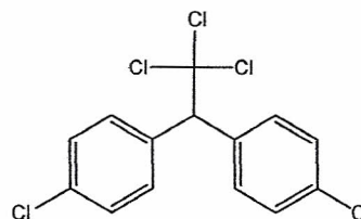
DDT
