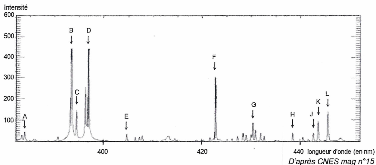
Document 4. Spectre d'émission atomique de la roche témoin réalisé par l'analyseur spectral de ChemCam dans le cadre du test de fonctionnement
