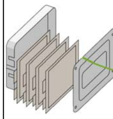
Composition d'un module (4 cellules en série)
