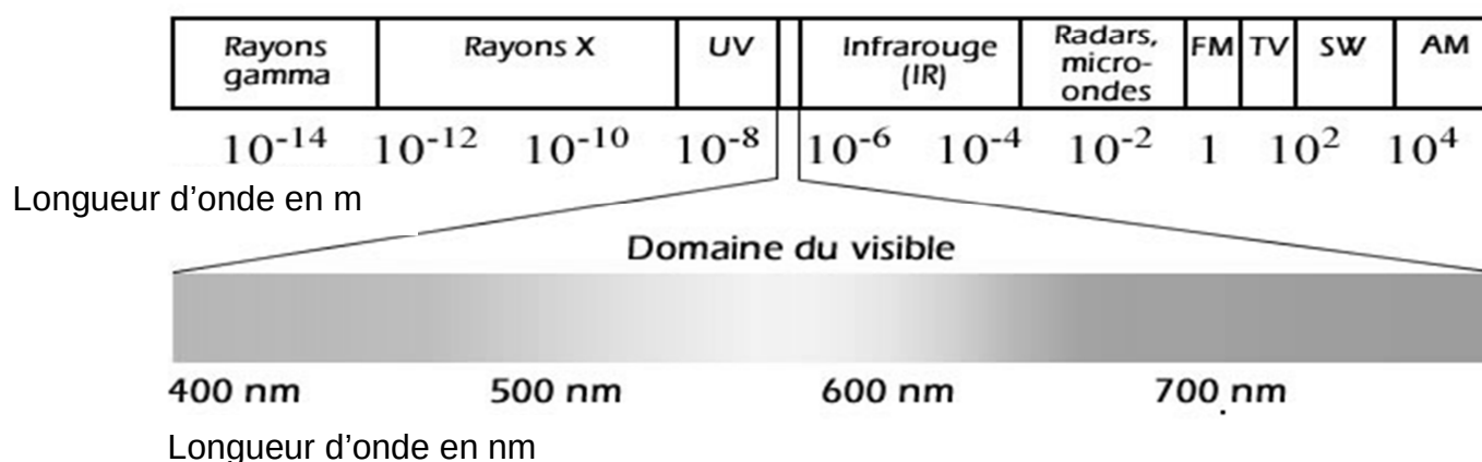
Document 10 Spectre des ondes électromagnétiques
